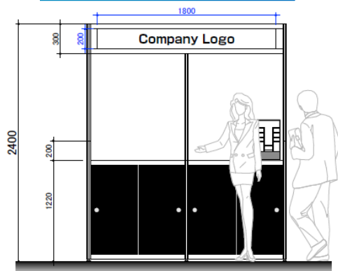
正面図
