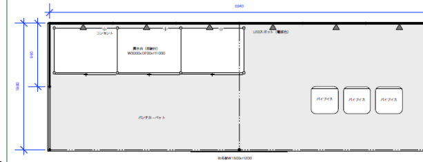
平面図
